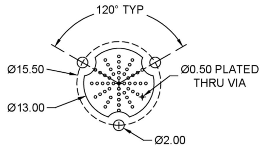
COPPER LAYER
