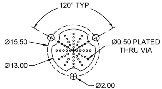
COPPER LAYER
