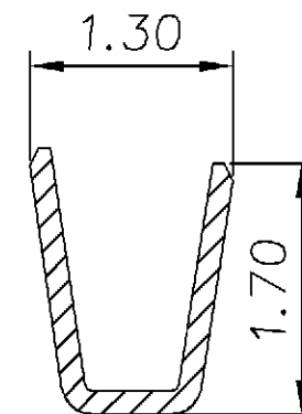
SEC A-A
