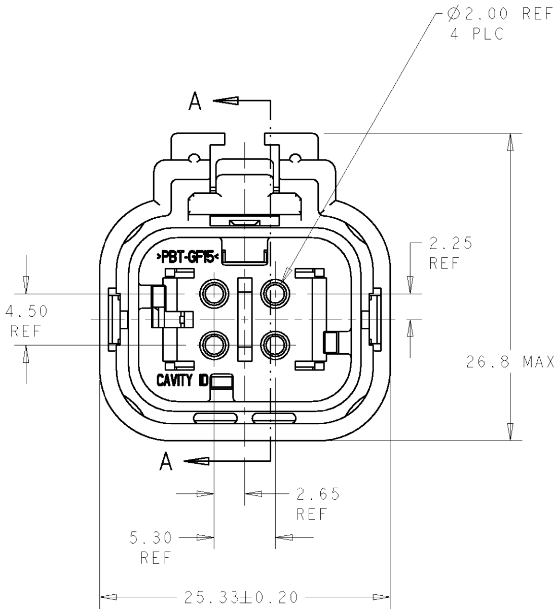
776487-1 SHOWN
