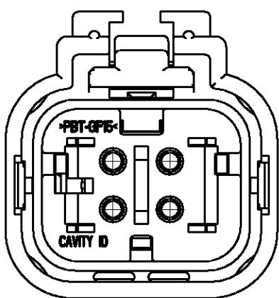
776487-3 SCALE 2:1
