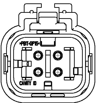
776487-4 SCALE 2:1
