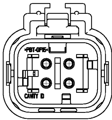
776487-2 SCALE 2:1
