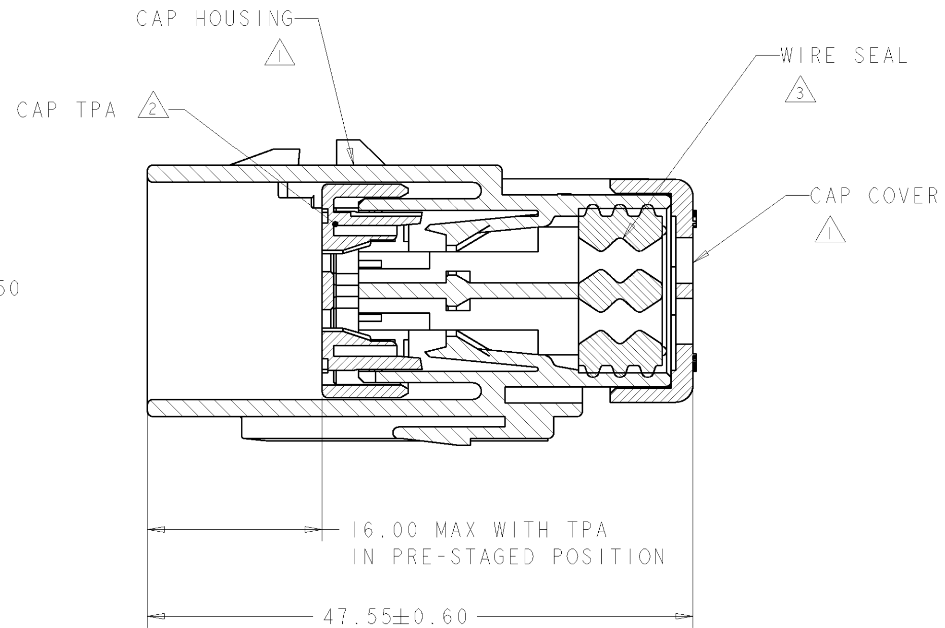
SECTION A-A
