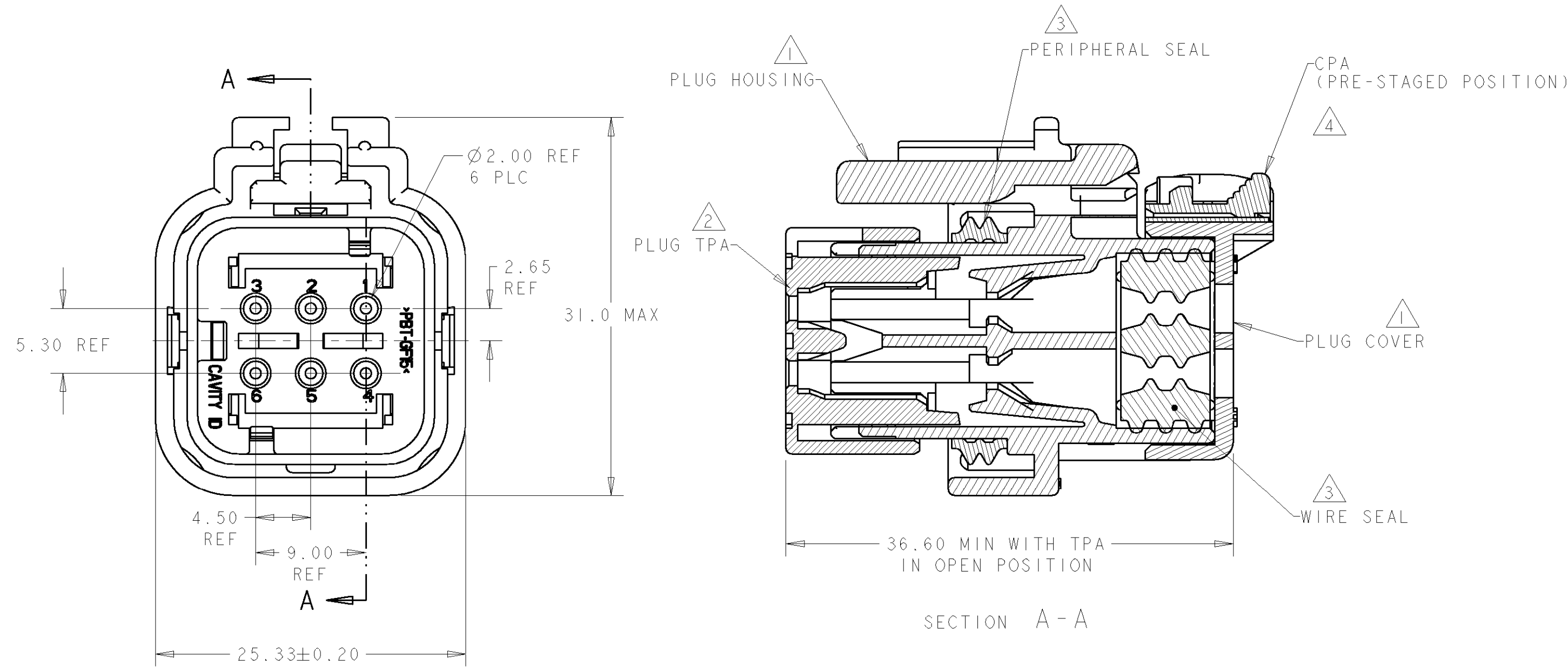
776531-1 SHOWN
