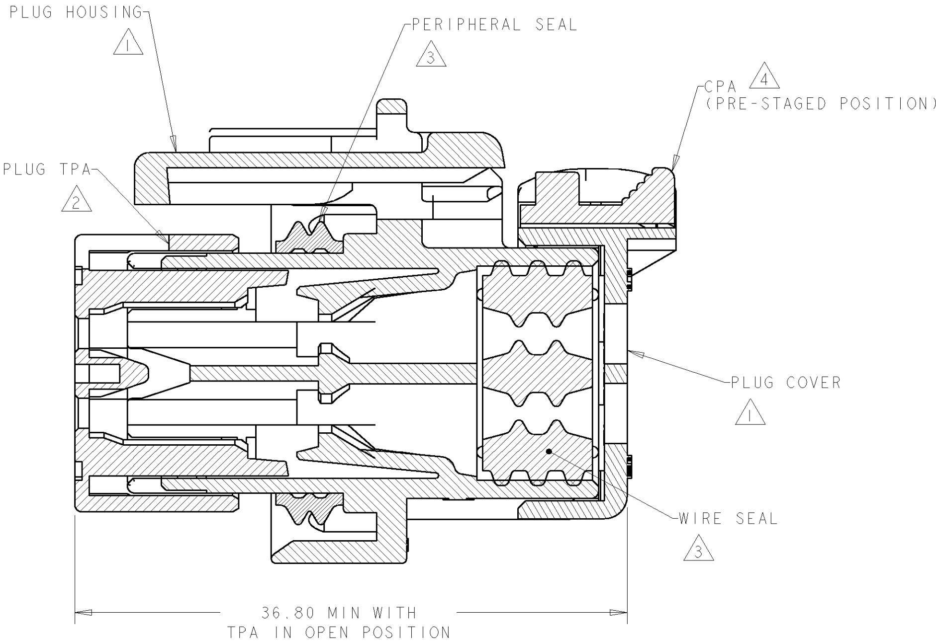
SECTION A-A
