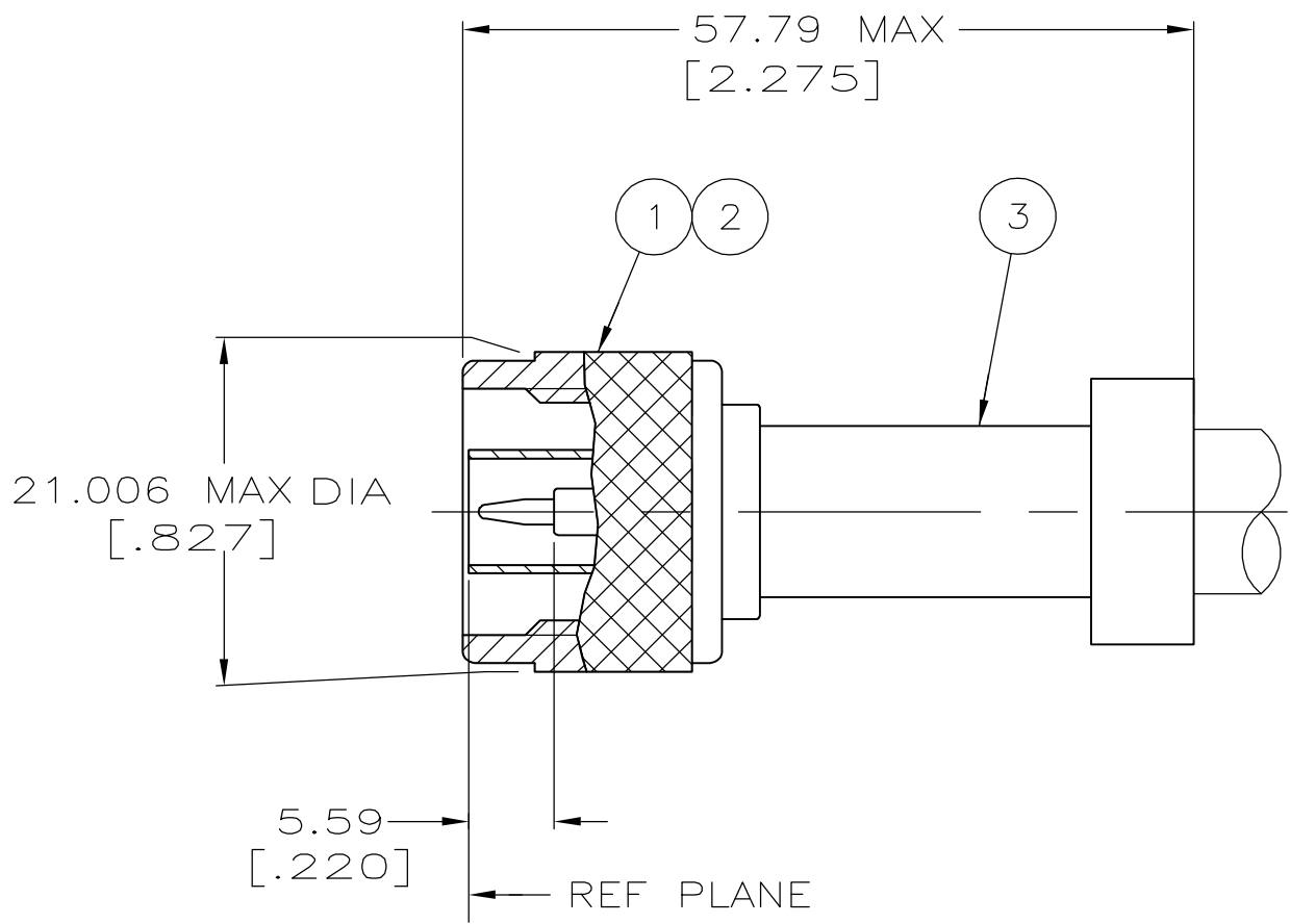
VIEW Y
