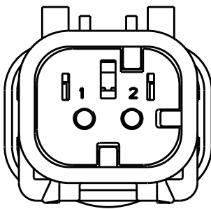
776428-2 SCALE 2:1 KEY B
