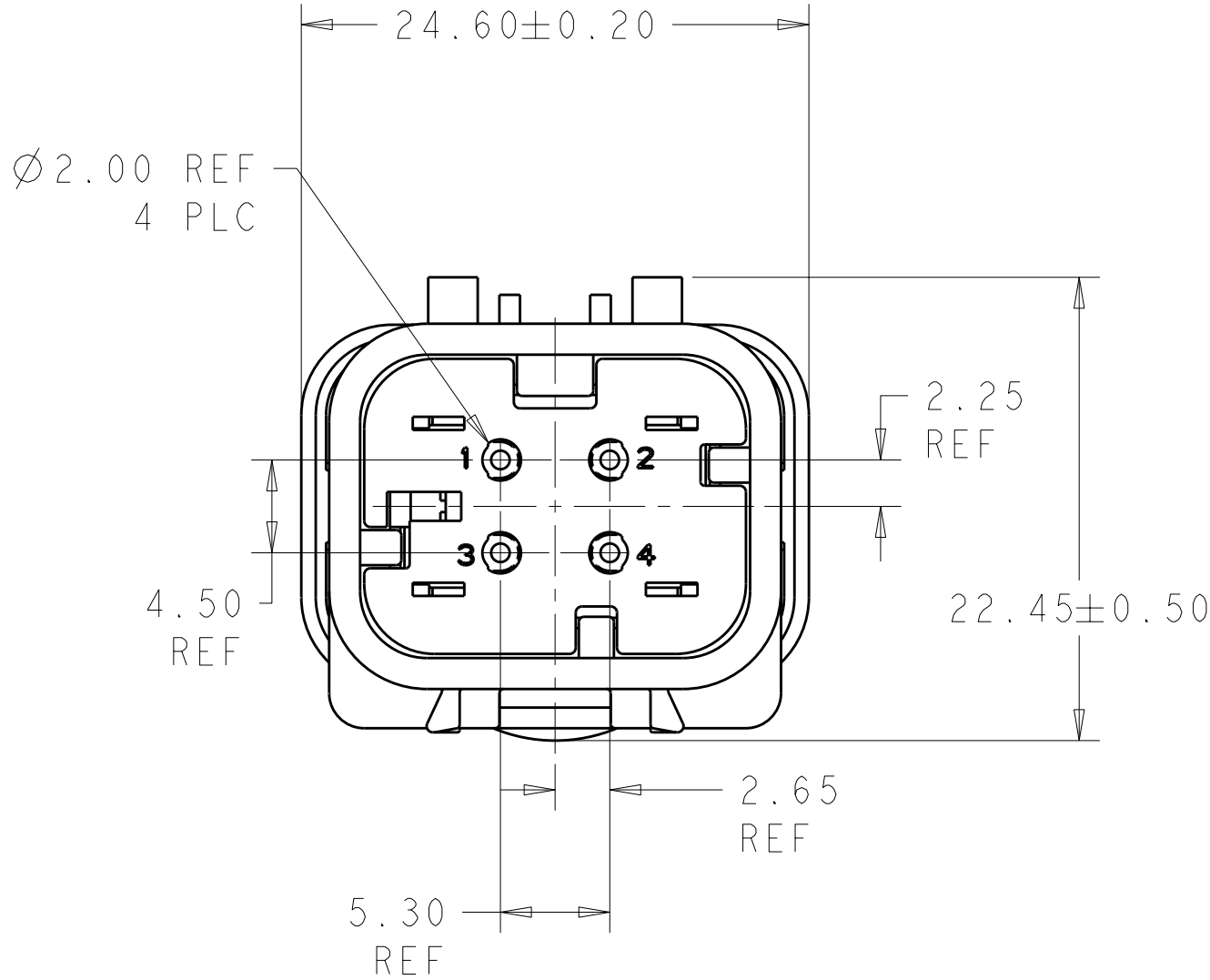
776536-1 SHOWN
