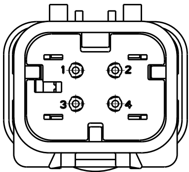
776536-3 SCALE 2:1
