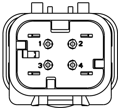
776536-2 SCALE 2:1
