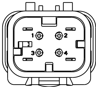
776536-4 SCALE 2:1
