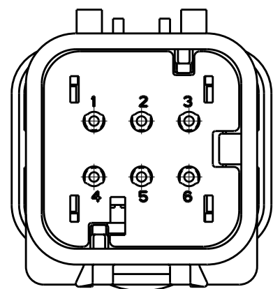
776537-2 SCALE 2:1
