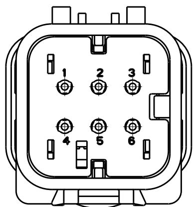
776537-3 SCALE 2:1
