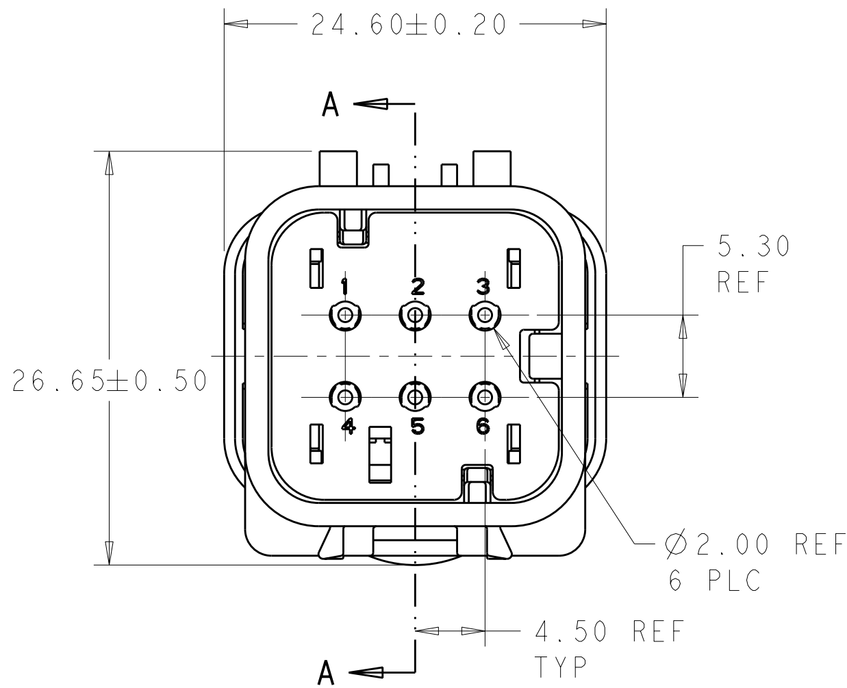
776537-1 SHOWN
