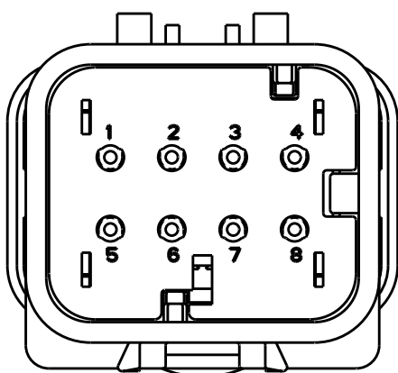
776538-4 SCALE 2:1
