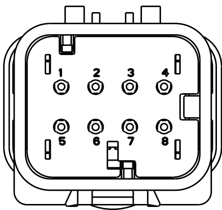
776538-3 SCALE 2:1
