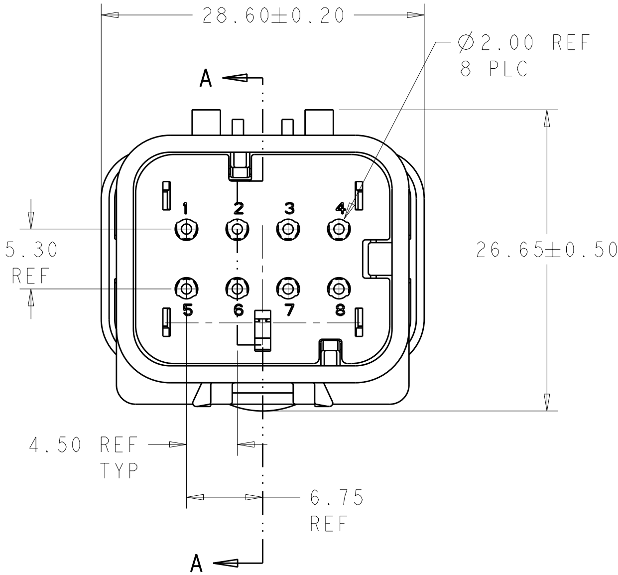
776538-1 SHOWN
