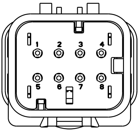
776538-2 SCALE 2:1
