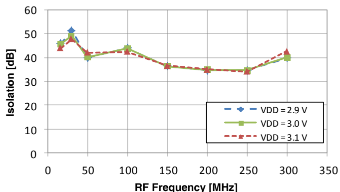
Figure 26. LO to IF Isolation vs V_{DD} (25 °C, -8 dBm LO Input, 110 MHz IF)
