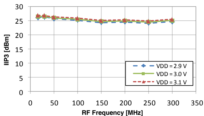
Figure 29. IIP3 vs V_{DD} (25 °C, -8 dBm LO Input, 110 MHz IF)
