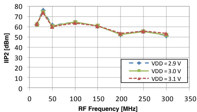
Figure 28. IIP2 vs V_{DD} (25 °C, -8 dBm LO Input, 110 MHz IF)
