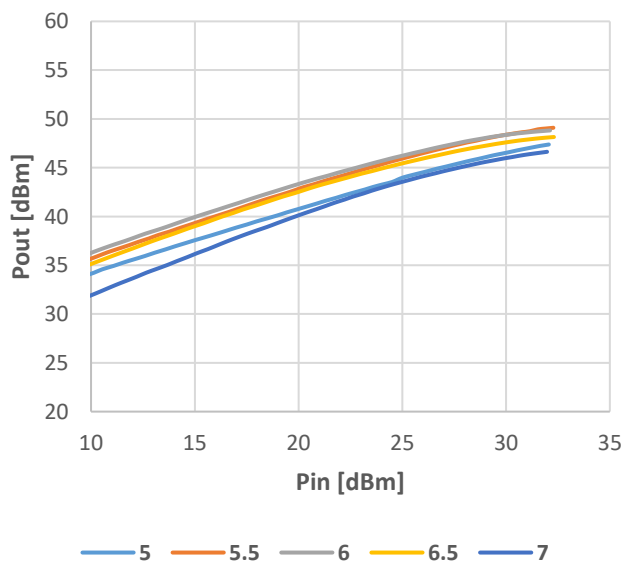
[28V] Pout vs. Pin
