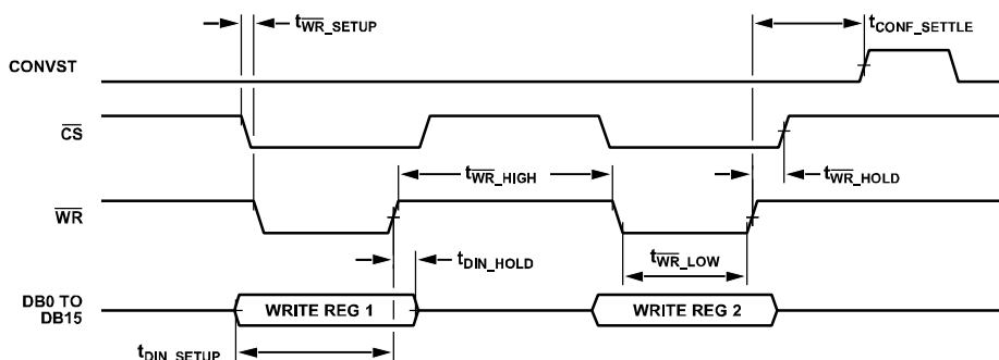
图5. 并行写入时序图
