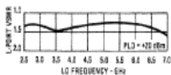
VSWR
