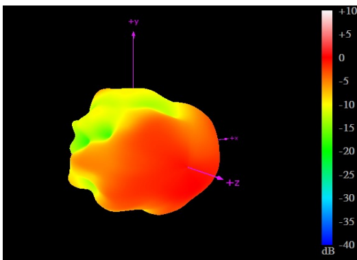
1710MHz
