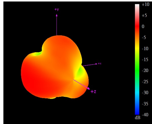
960MHz
