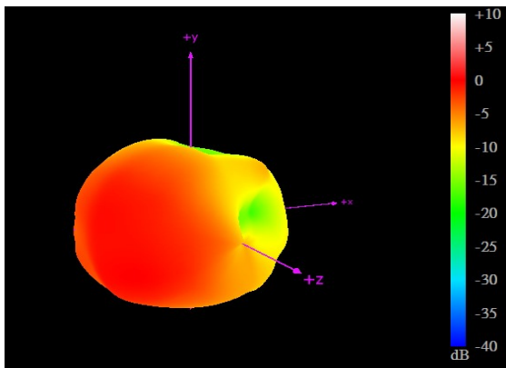
1710MHz
