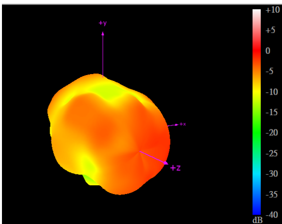
2690MHz
