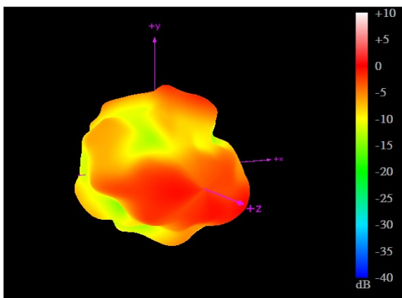
2690MHz
