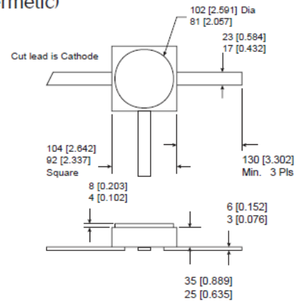
H30 (hermetic)
